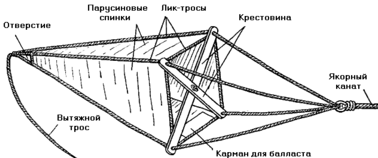
Рис. 117. Плавучий якорь
