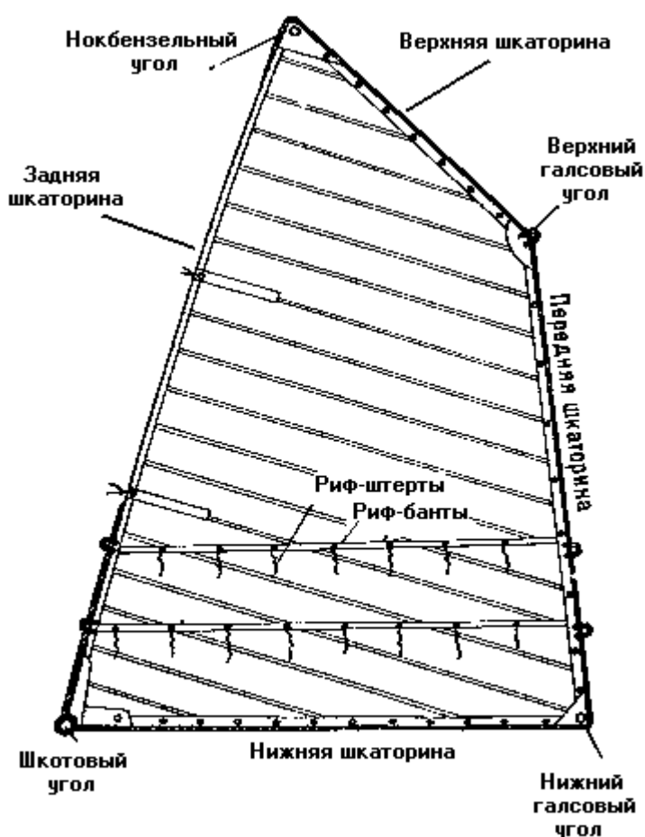
Рис. 36. Гафельный грот и его части
