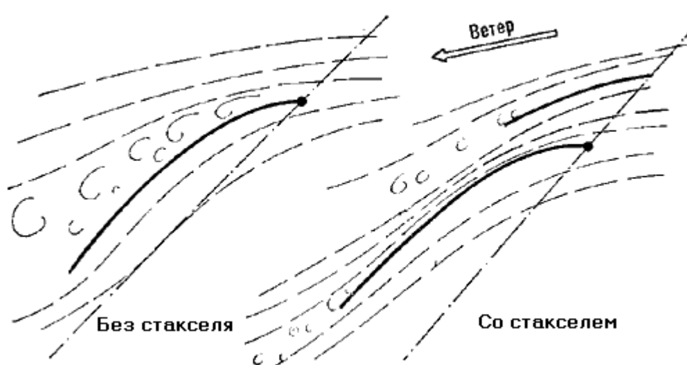
Рис. 97. Работа стакселя
