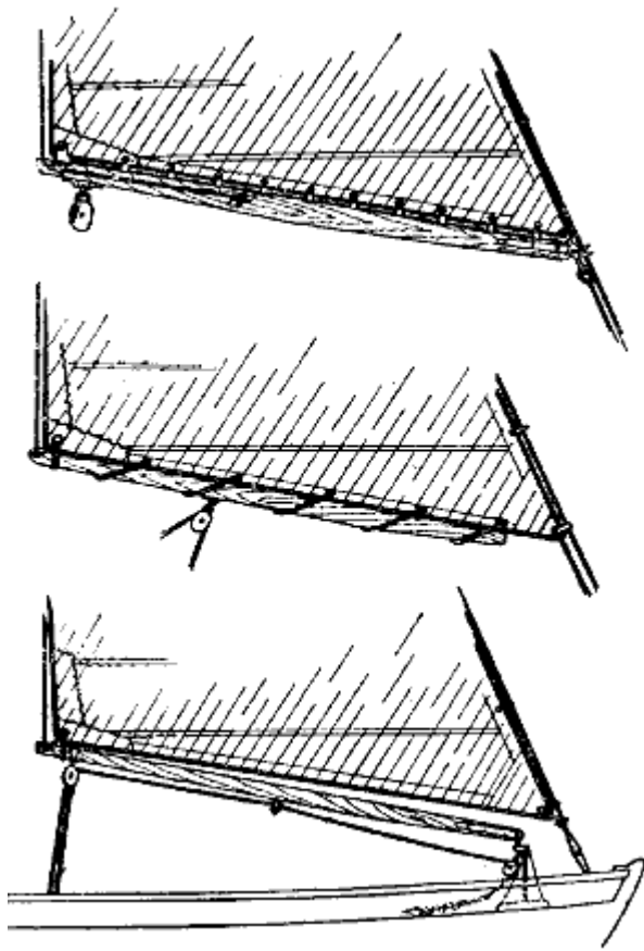
Рис. 43. Рейки стакселей
