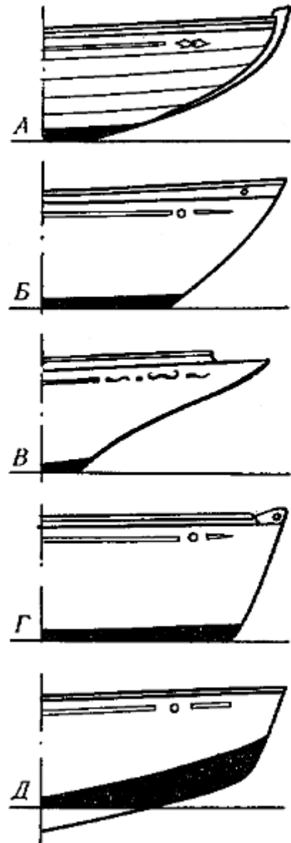
Рис. 11. Формы носовых частей: А — ложкообразный штевень; Б — современный наклонный штевень; В — клипер-штевень; Г — прямой штевень; Д — транце вый нос (форшпигель) швертбота «Кадет»
