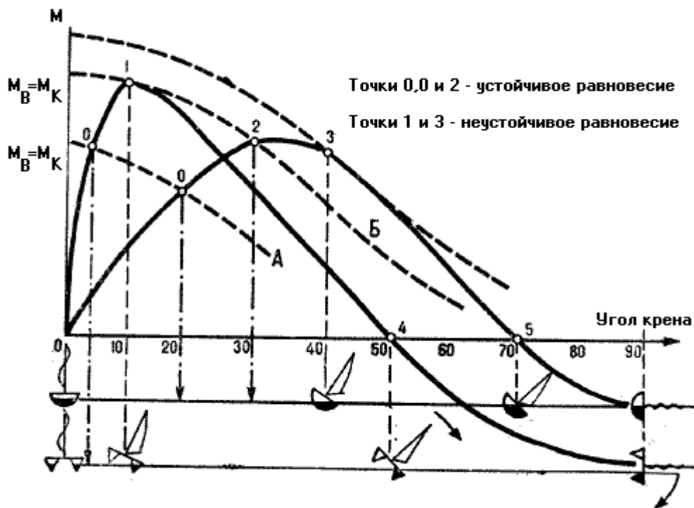
Рис. 82. Остойчивость швертбота и катамарана при действии ветра на паруса
