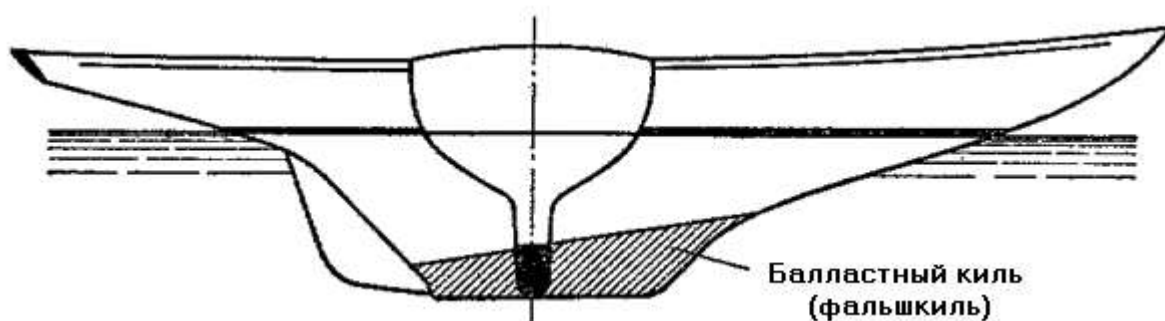
Рис. 4. Килевая яхта
