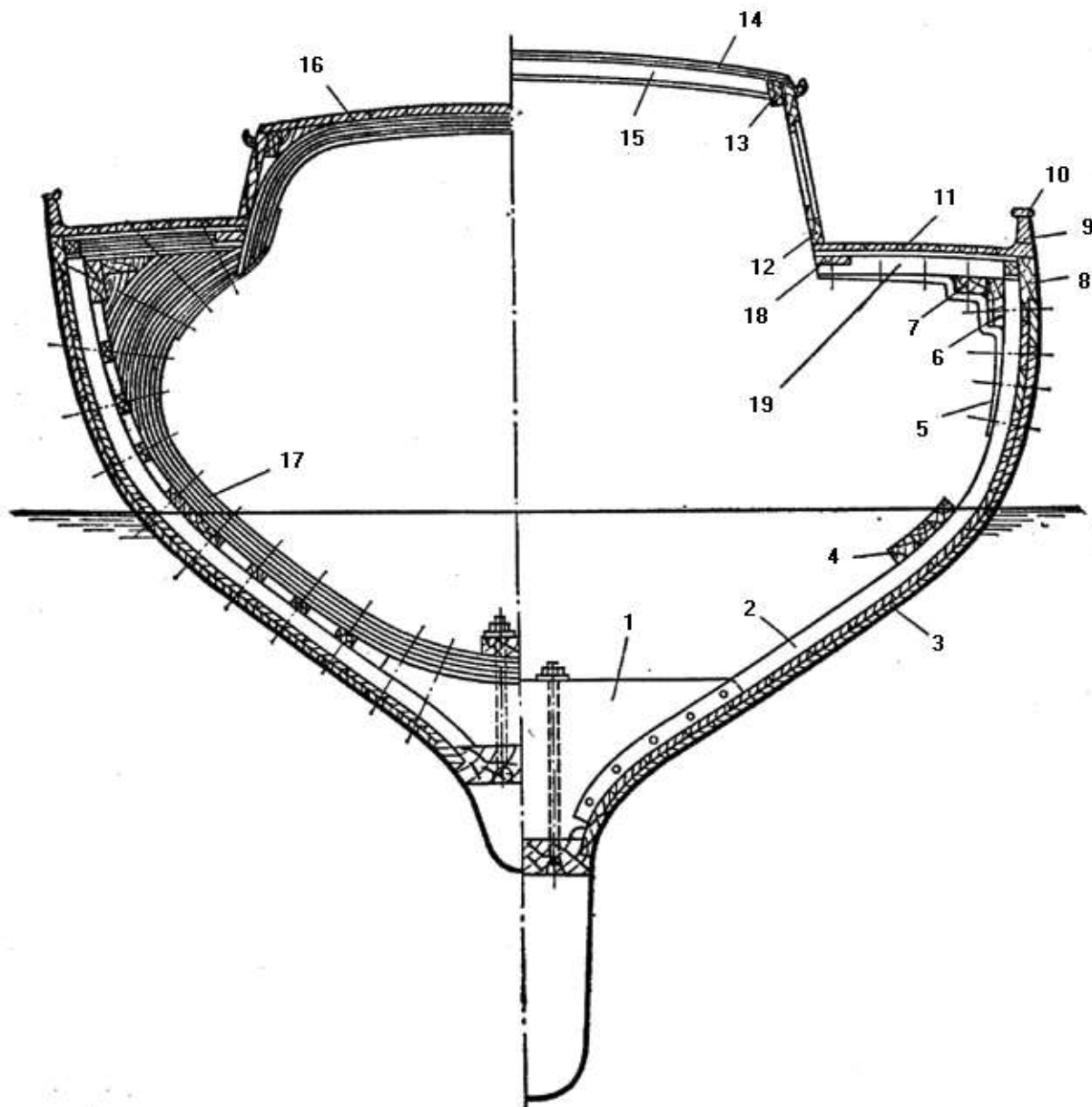
Рис. 27. Поперечный разрез деревянной кругло-шпангоутной яхты: 1 — флор; 2 — шпангоут; 3 — двойная продольная обшивка; 4 — скуловой стрингер; 5 — висячая кница; 6 — привальный брус; 7 — шельф; 8 — ширстрек; 9 — фальшборт; 10 — планширь; 11 — палубный настил; 12 — комингс рубки; 13 — шельф; 14, 16 — крыша рубки; 15 — бимс; 17 — усиленный рамный шпангоут; 18 — карленгс; 19 — полубимс
