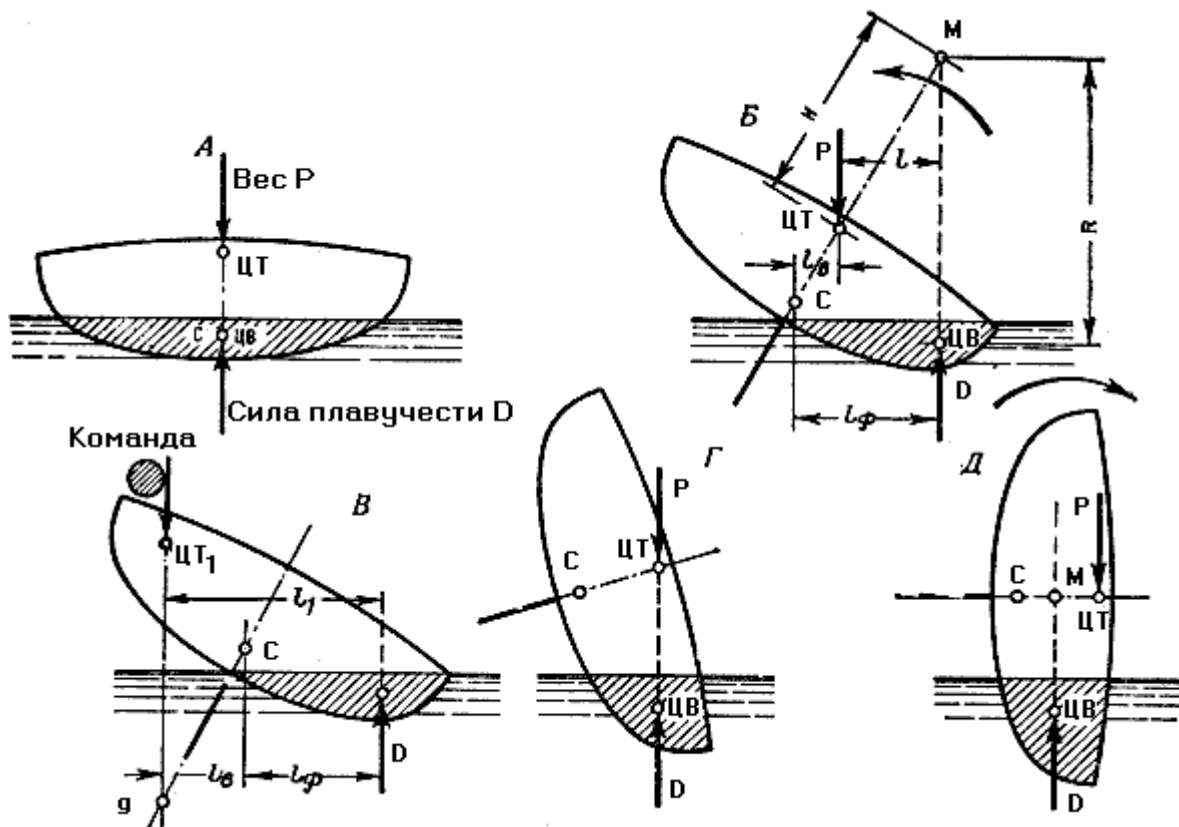
Рис. 78. Остойчивость швертбота
