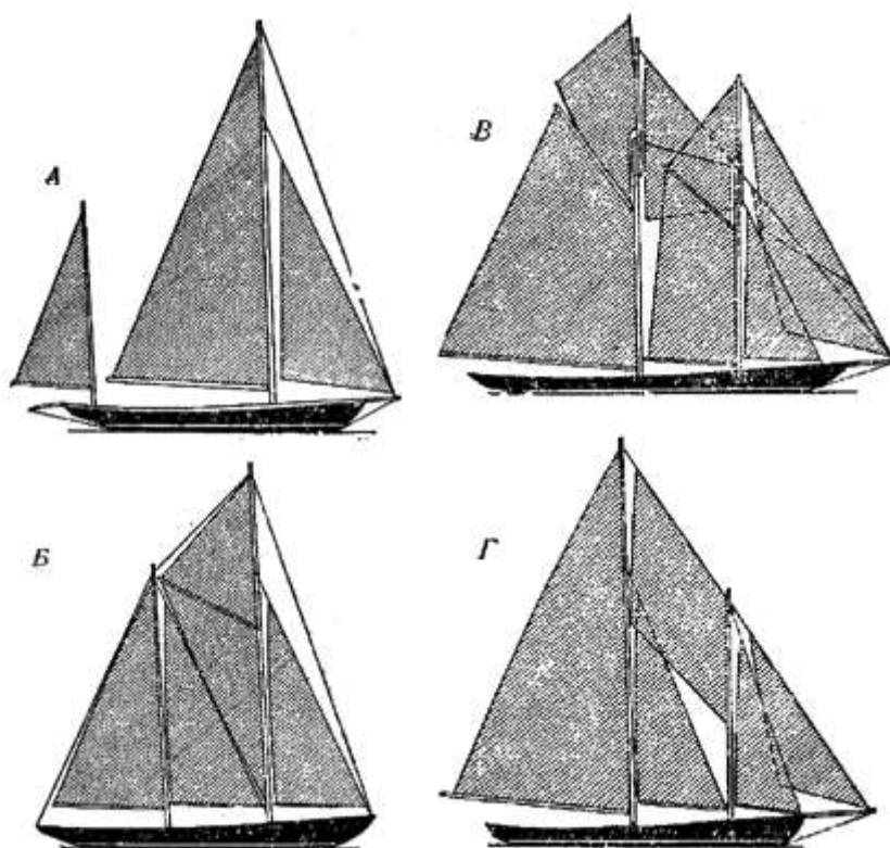
Рис. 15. Двухмачтовые яхты. A — бермудский иол; б — стаксельный кэч. B — гафельная шхуна; Г — бермудская стаксельная шхуна
