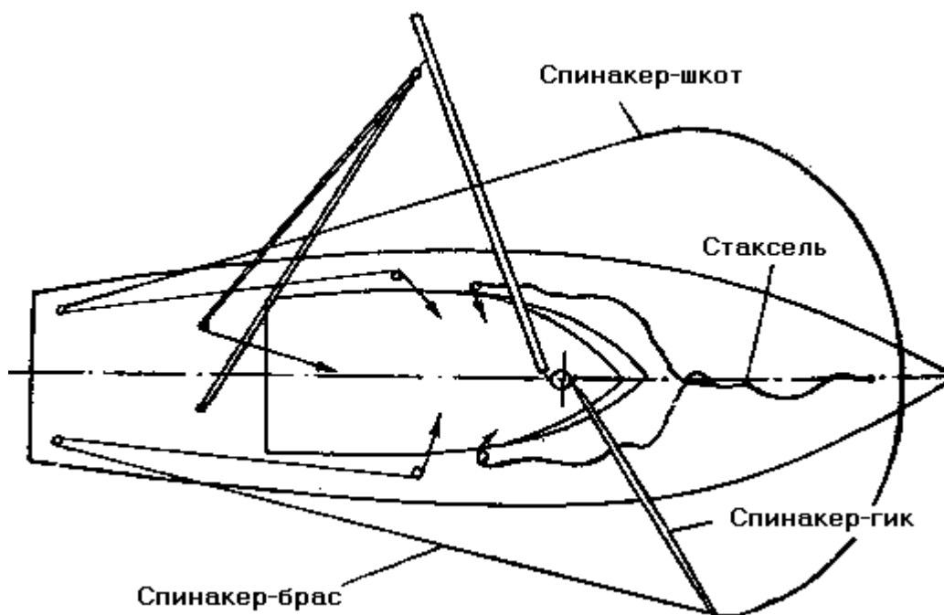
Рис. 48. Такелаж спинакер-гика
