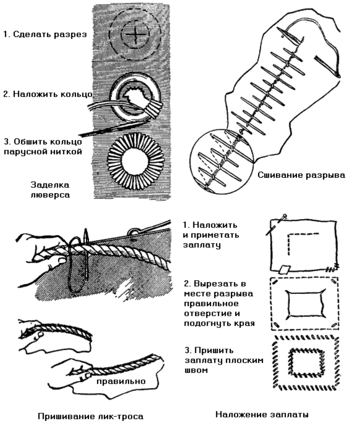
Рис. 72. Ремонт парусов
