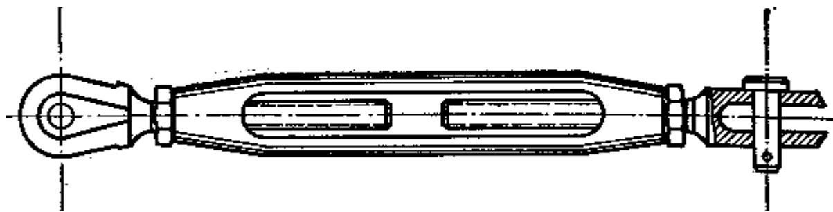
Рис. 40. Винтовой талреп
