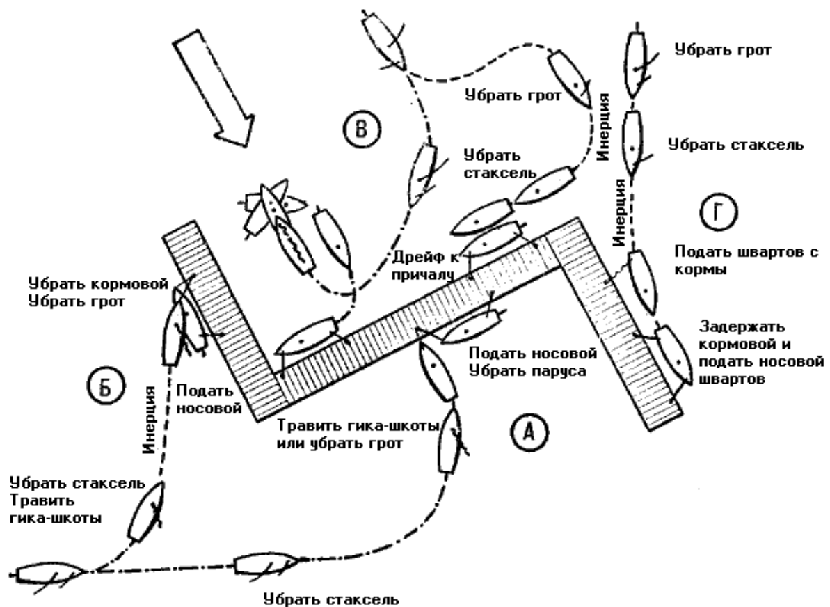
Рис. 125. Как подойти к причалу:
