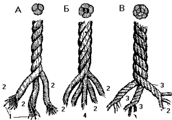
Рис. 55. Растительные тросы: А—трехпрядный тросовой работы; Б—четырепрядный тросовой работы с сердечником; В — кабельной работы; 1 — каболки; 2 — пряди; 3 — стренди; 4 — сердечник.
