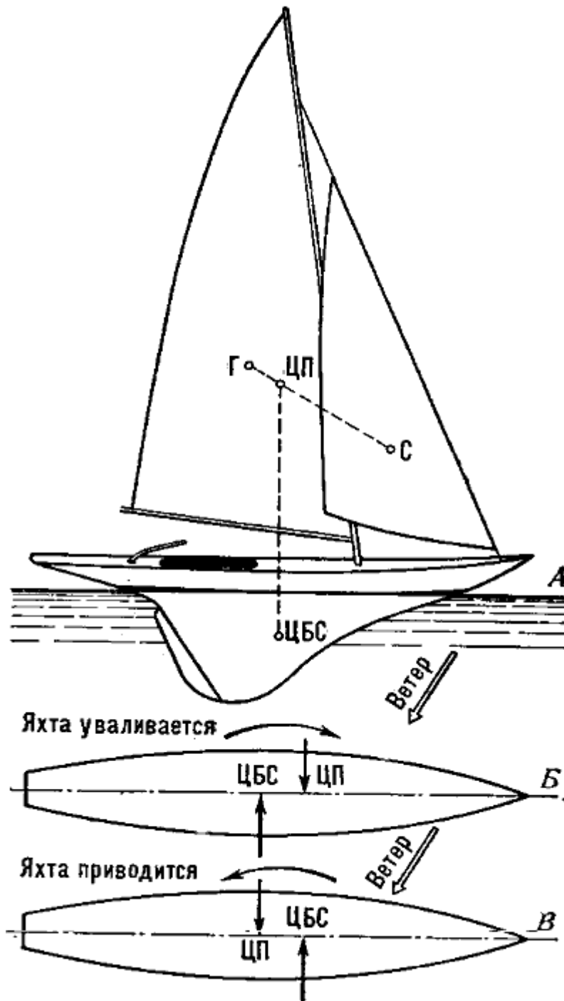
Рис. 99. Центровка яхты
