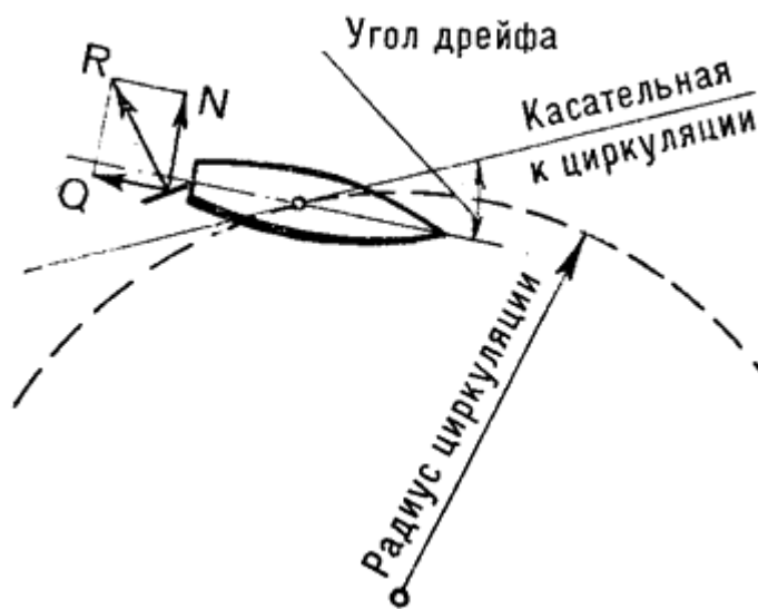
Рис. 83. Схема действия руля
