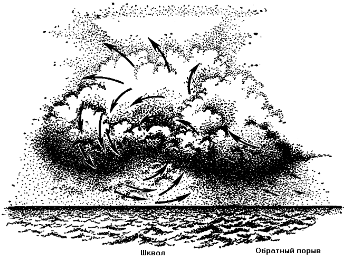
Рис 121 Схема циркуляции воздуха под шквальным облаком
