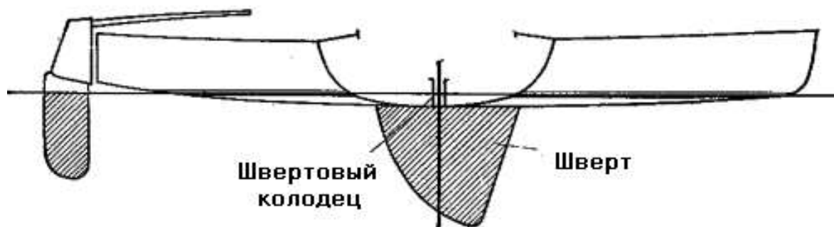
Рис. 5. Швертбот
