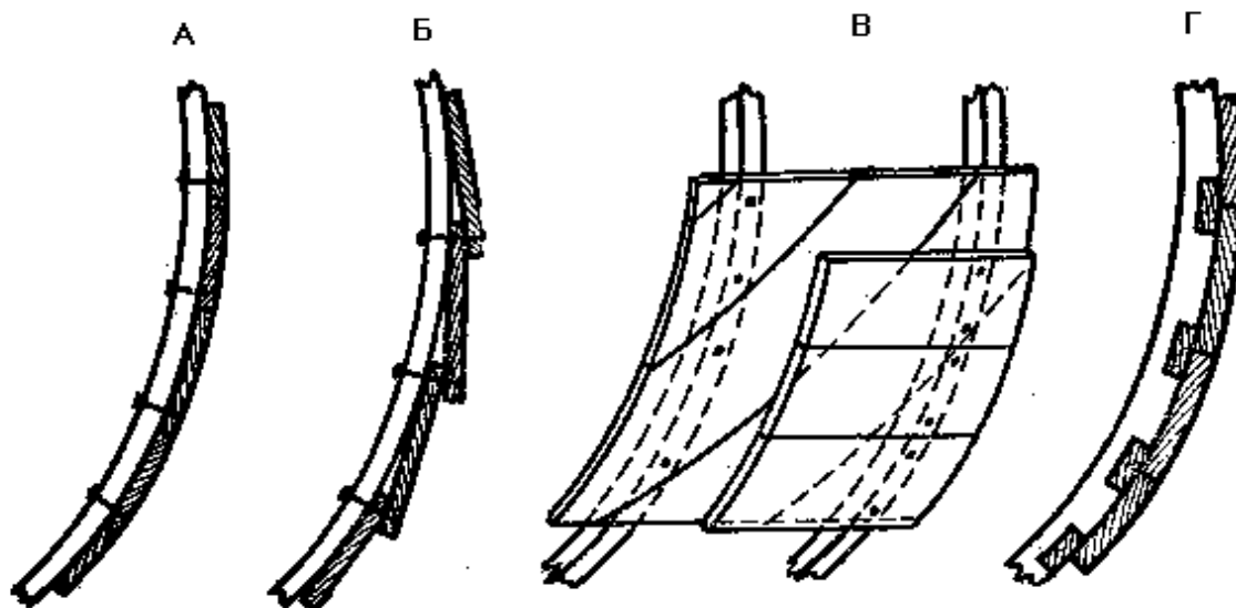
Рис. 29. Виды обшивки:
