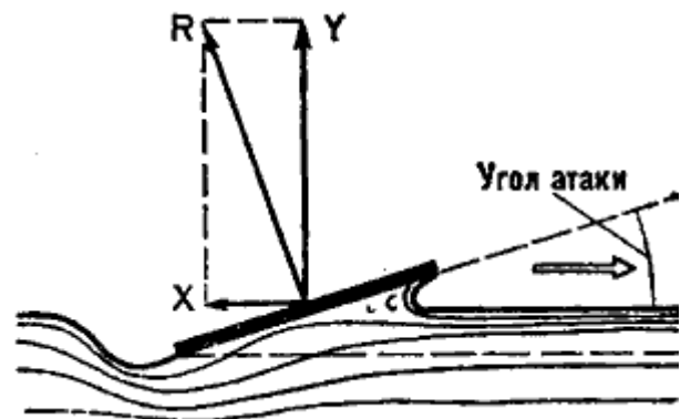
Рис. 87. Давление воды на движущуюся плоскую пластинку
