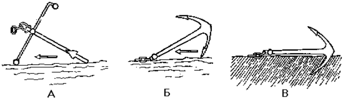
Рис. 53. Работа адмиралтейского якоря
