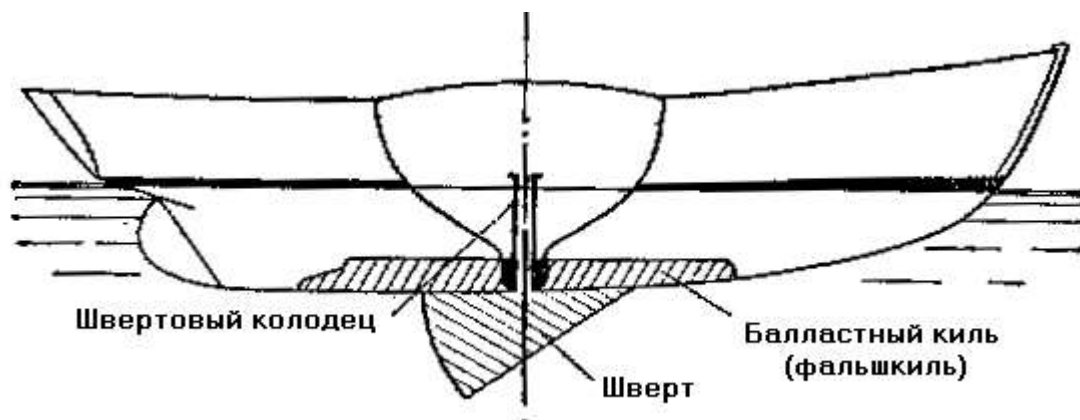
рис. 6. Яхта-компромисс
