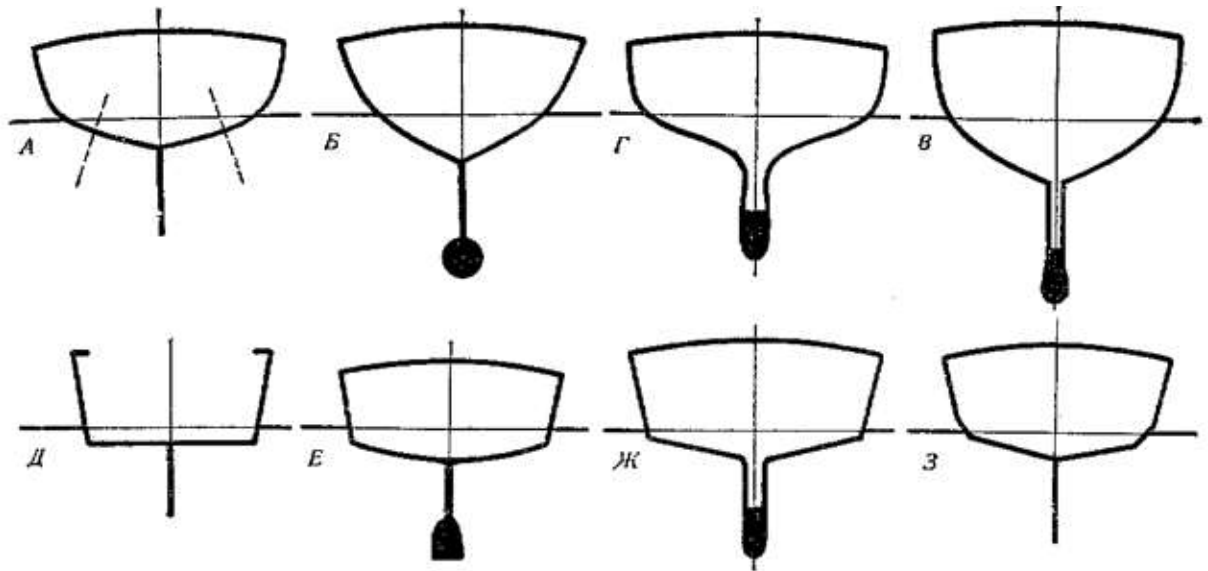
Рис. 9. Формы мидель-шпангоутов.
