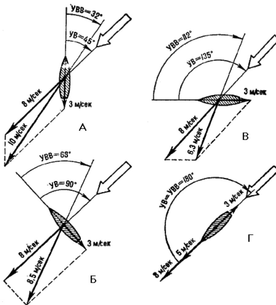
Рис. 90. Вымпельный ветер на разных курсах
