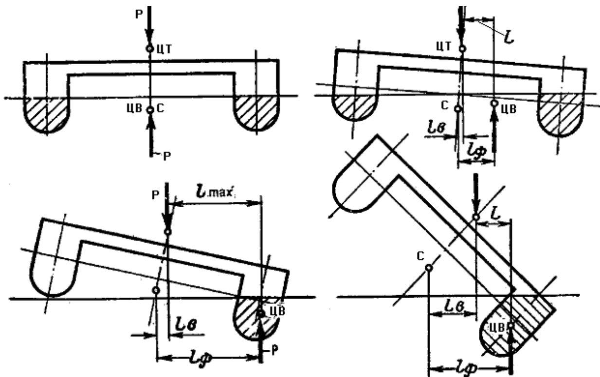
Рис. 81. Остойчивость катамарана
