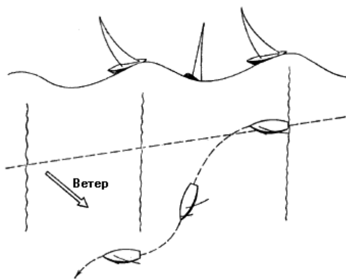
Рис. 116. Управление яхтой на волне
