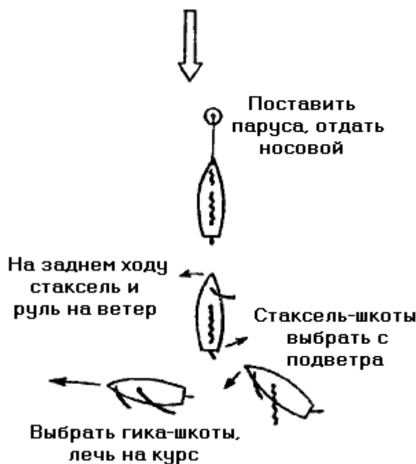
Рис. 123. Отход от бочки или причала на заднем ходу, когда за кормой есть место
