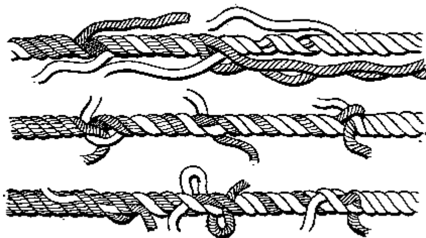
Рис. 64. Лонгоспесень (длинный сплесень)
